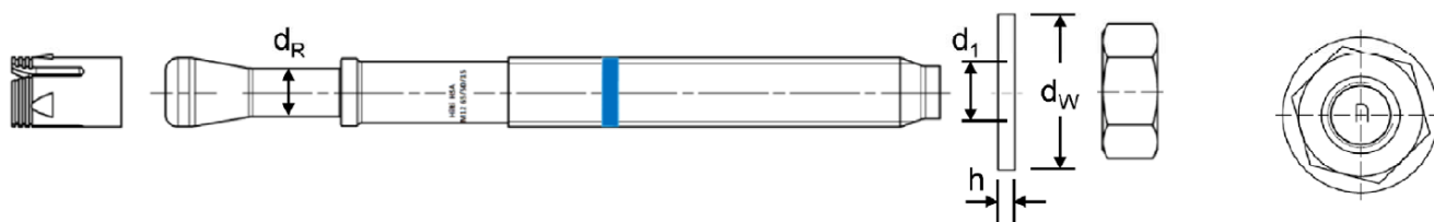
Rysunek A1: Metalowa kotwa rozporowa Hilti HSA, HSA-F, HSA-R2, HSA-R
