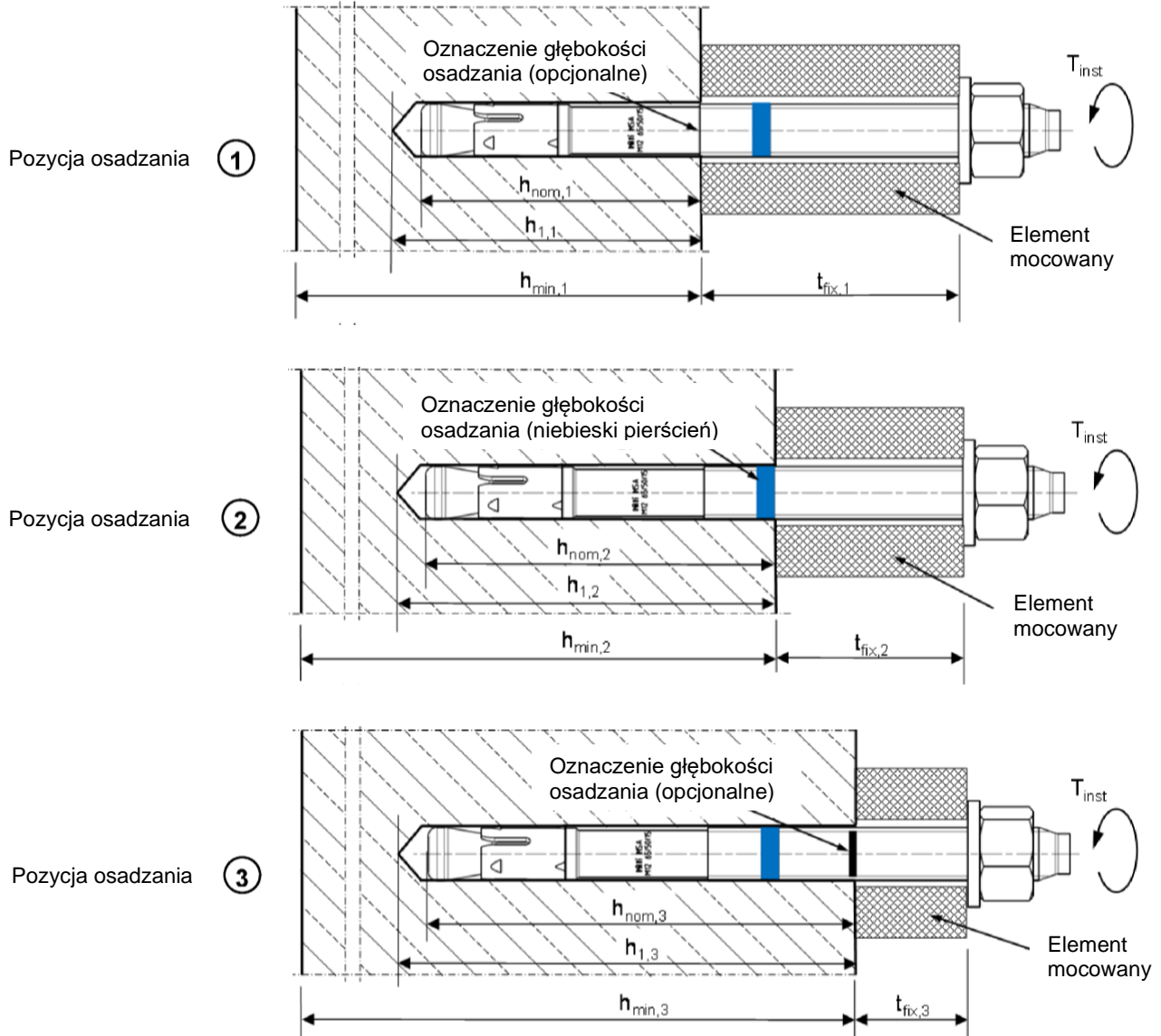
Rysunek B1: Stała długość kotwy dla różnych grubości mocowanego elementu t_{fix} oraz odpowiednich pozycji osadzenia
