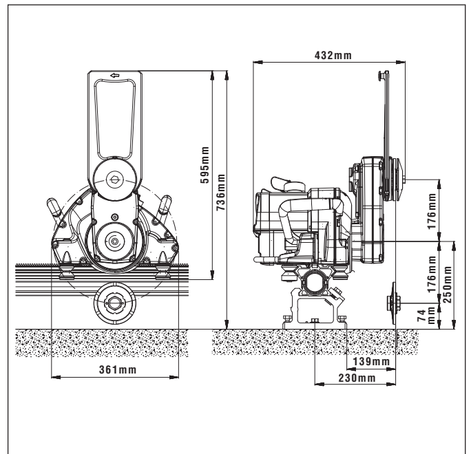
Κύριες διαστάσεις του DS TS20-E (σε χιλ.)
